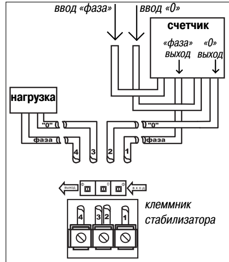
Рис. 17. Схема установки
