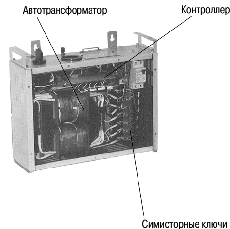
Рис. 8. Устройство стабилизатора
