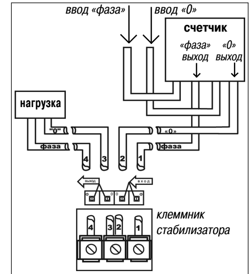
Рис. 17. Схема установки
