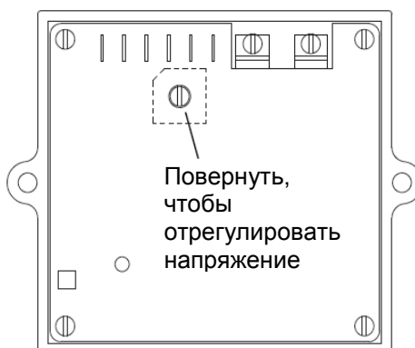
Рисунок 2.2 – Потенциометр регулировки напряжения
