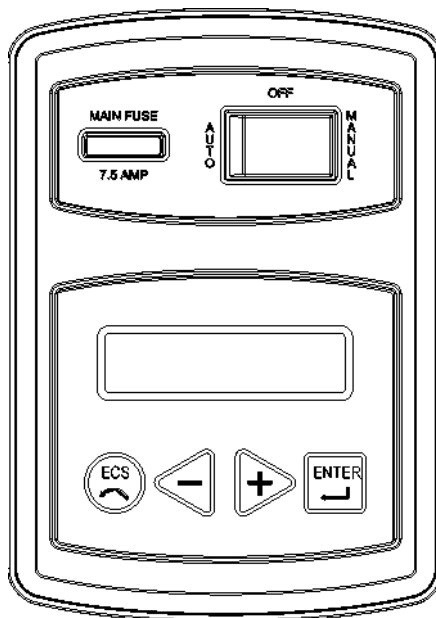
Рисунок 3.2 – Панель управления 10/12/14/16/17 и 20кВт генераторов
