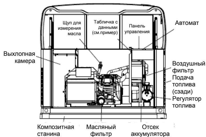
Рисунок 1.1 – 8кВт, одноцилиндровый двигатель GH-410 (со съёмной дверцей)
