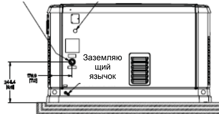
ВИД СЗАДИ
