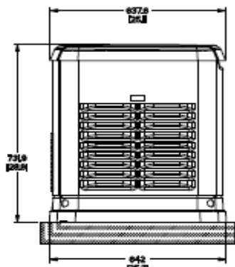
ВИД СЛЕВА
