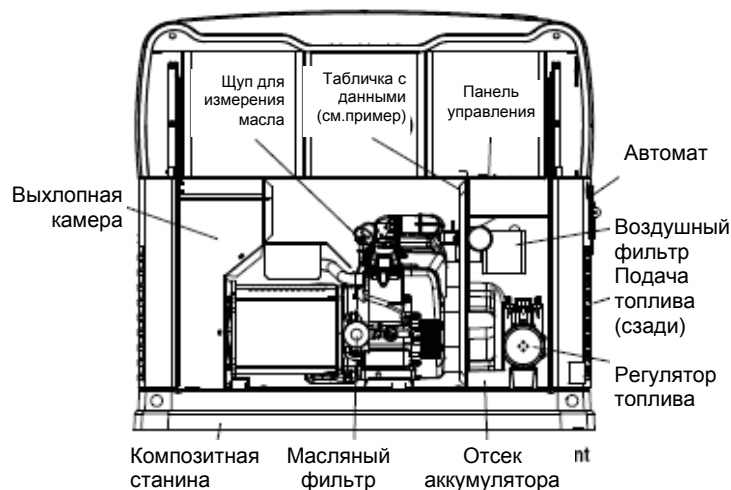
Рисунок 1.2 – 10кВт, двухцилиндровый V-образный двигатель GT-530 (со съёмной дверцей)
