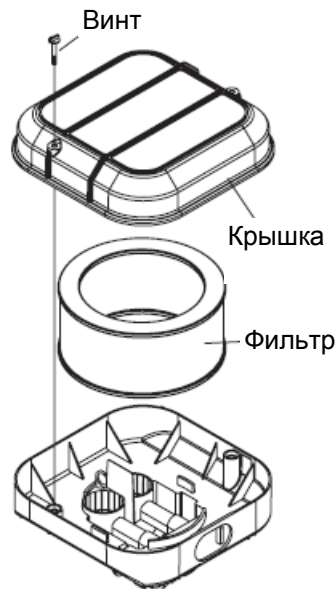
Рисунок 4.5 — Воздухоочиститель двигателя на моделях 12, 14, 16, 17 и 20кВт
