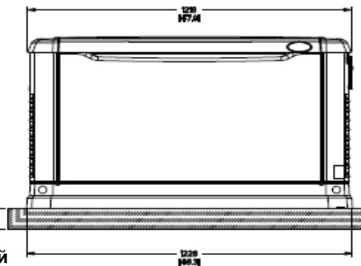
ВИД СПЕРЕДИ
