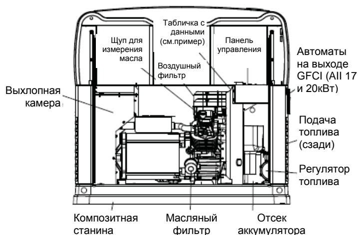
Рисунок 1.3 – 12, 14, 16, 17 и 20кВт, двухцилиндровый V-образный двигатель GT-990/GT-999 (со съемной дверцей)
