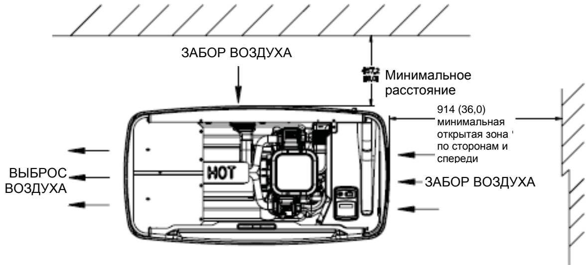
ВИД СВЕРХУ
