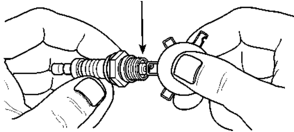
Рисунок 4.8 – Установка зазора между электродами свечи Установить зазор между электродами свечи на 0,76мм (0,030 дюйма) для моделей 8, 10 и 20кВт; и 1,02 мм (0,040 дюйма) для моделей 12, 14, 16 и 17кВт
