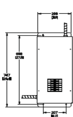
Передаточный ключ 8 – 17 кВт (если есть в поставке)
